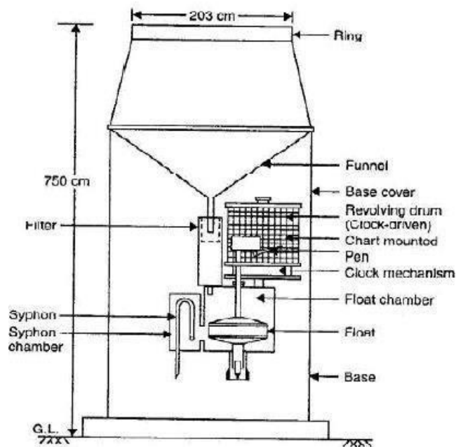
FIG: SIPHON RAINGAUGE
